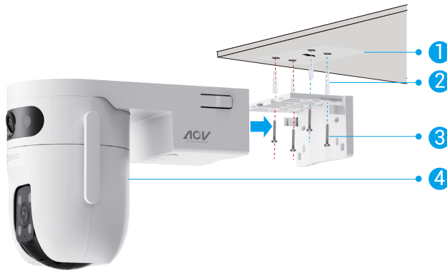
그림 1 천장 장착
