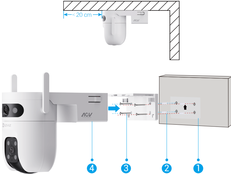
그림 2 벽 장착
