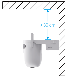
그림 2 벽 장착
